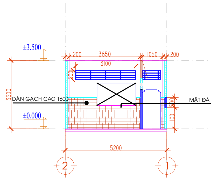
MẶT CẮT 3-3 HOÀN CHỈNH
