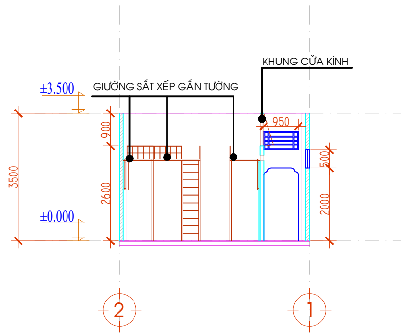
MẶT CẮT 2-2 HOÀN CHỈNH
