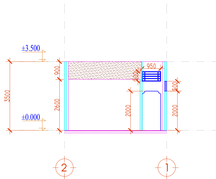
MẶT CẮT 2-2 HIỆN TRẠNG
