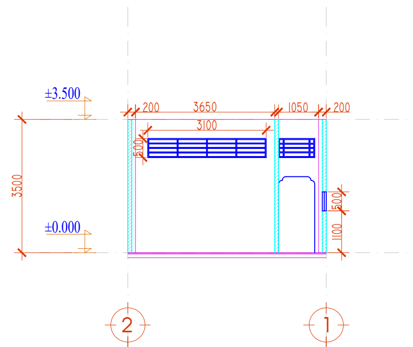
MẶT CẮT 3-3 HIỆN TRẠNG
