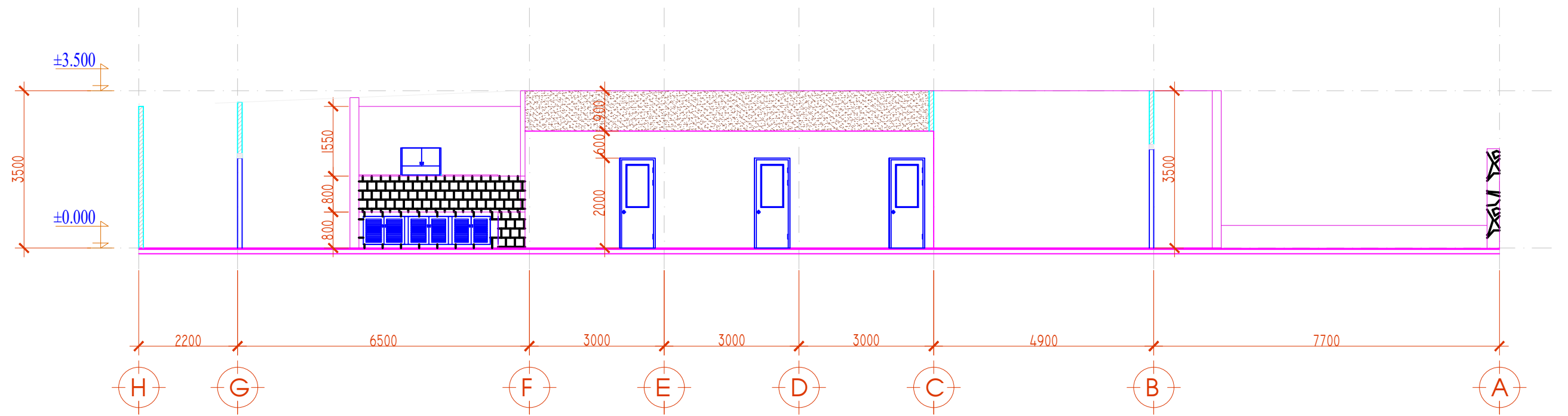
MẶT CẮT 1-1 HOÀN CHỈNH
